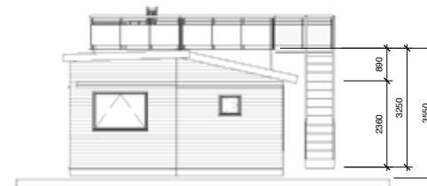
2 Norr 1 : 100
