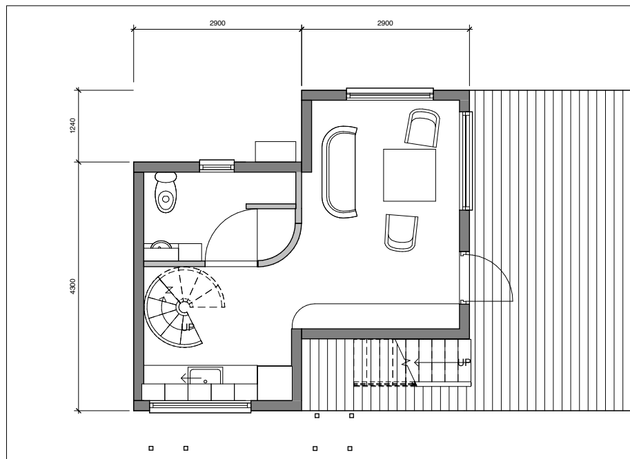
1 Plan 1 1-50 1 : 50
