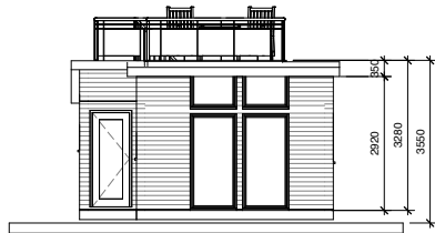
1 Öst 1 : 100
