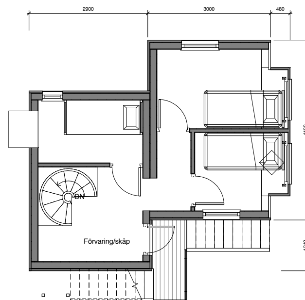
2 Plan 2 1-50 1 : 50
