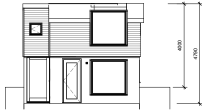
1 Öst 1 : 100
