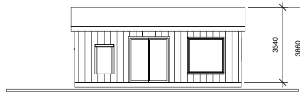
4 Syd 1 : 100
