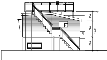
3 Syd 1 : 100
