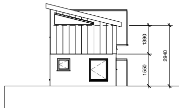
3 Väst 1 : 100
