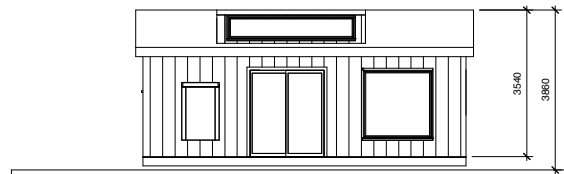
4 Syd 1 : 100
