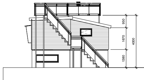
3 Syd 1 : 100
