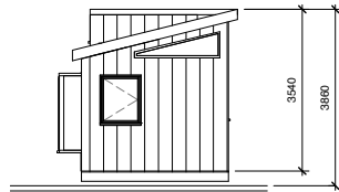
1 Öst 1 : 100
