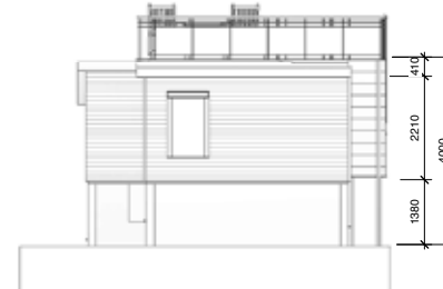
4 Väst 1 : 100
