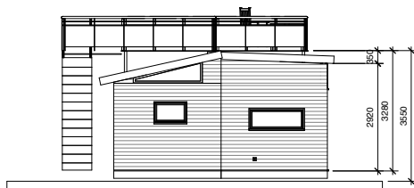
3 Syd 1 : 100
