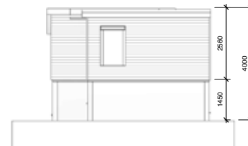
4 Väst 1 : 100
