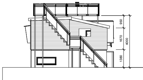
3 Syd 1 : 100
