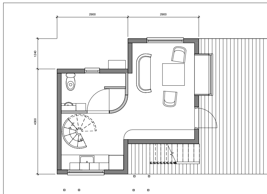
1 Plan 1 1-50 1 : 50
