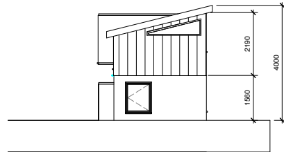
1 Öst 1 : 100
