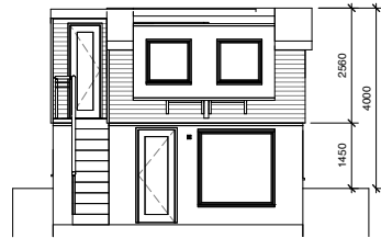
1 Öst 1 : 100
