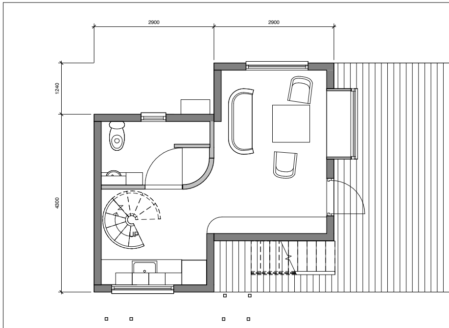
1 Plan 1 1-50 1 : 50
