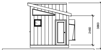
3 Väst 1 : 100
