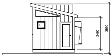
3 Väst 1 : 100
