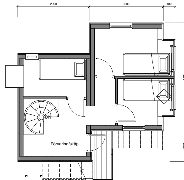
2 Plan 2 1-50 1 : 50
