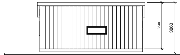
2 Norr 1 : 100
