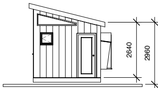
3 Väst 1 : 100
