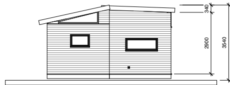
3 Syd 1 : 100
