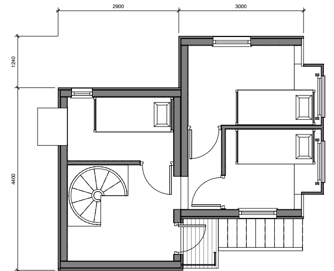
2 Level 2 1to1 1 : 50
