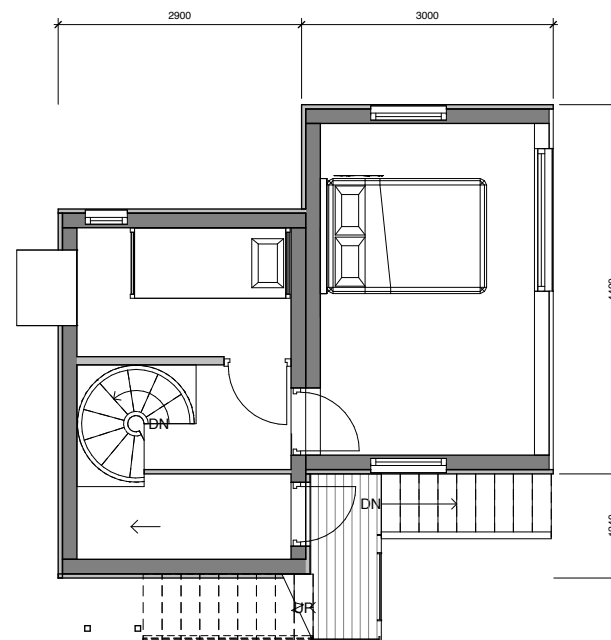
2 Plan 2 1-50 1 : 50
