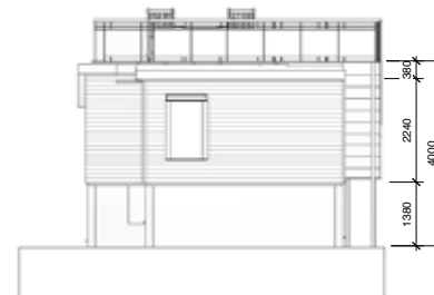
4 Väst 1 : 100
