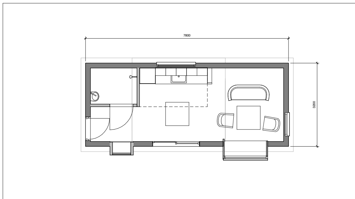
1 Plan 1-50 1 : 50
