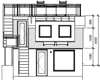
1 Öst 1 : 100
