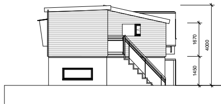
3 Syd 1 : 100
