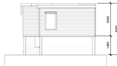
4 Väst 1 : 100
