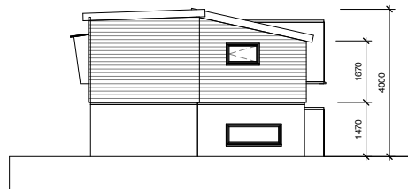
3 Syd 1 : 100
