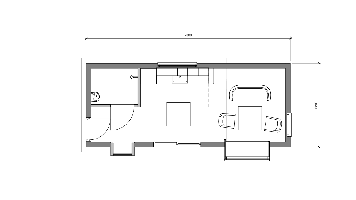
1 Plan 1-50 1 : 50
