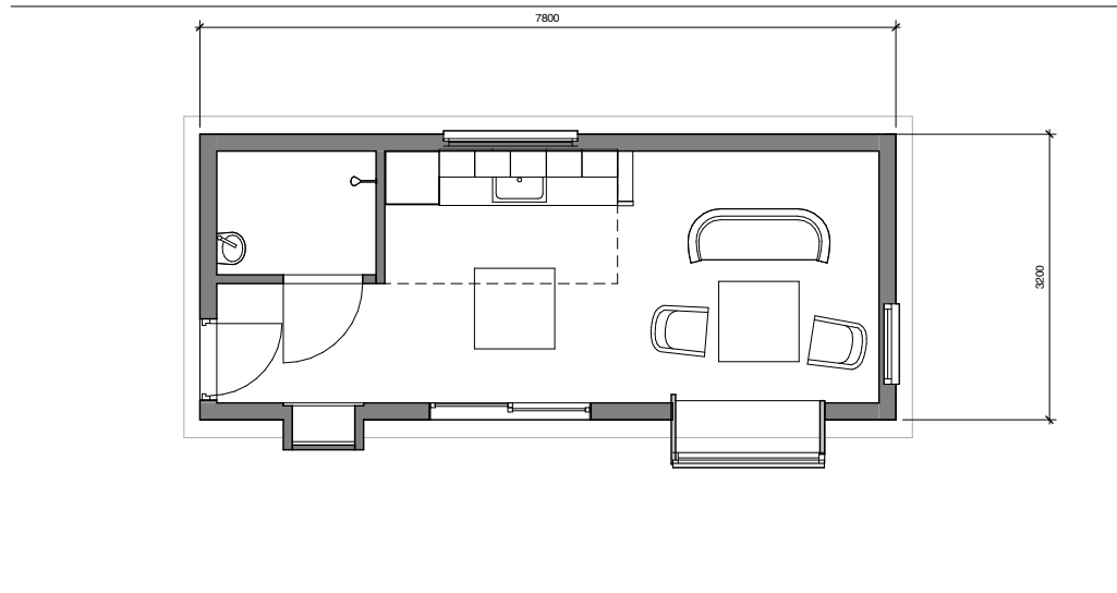
1 Plan 1-50 1 : 50
