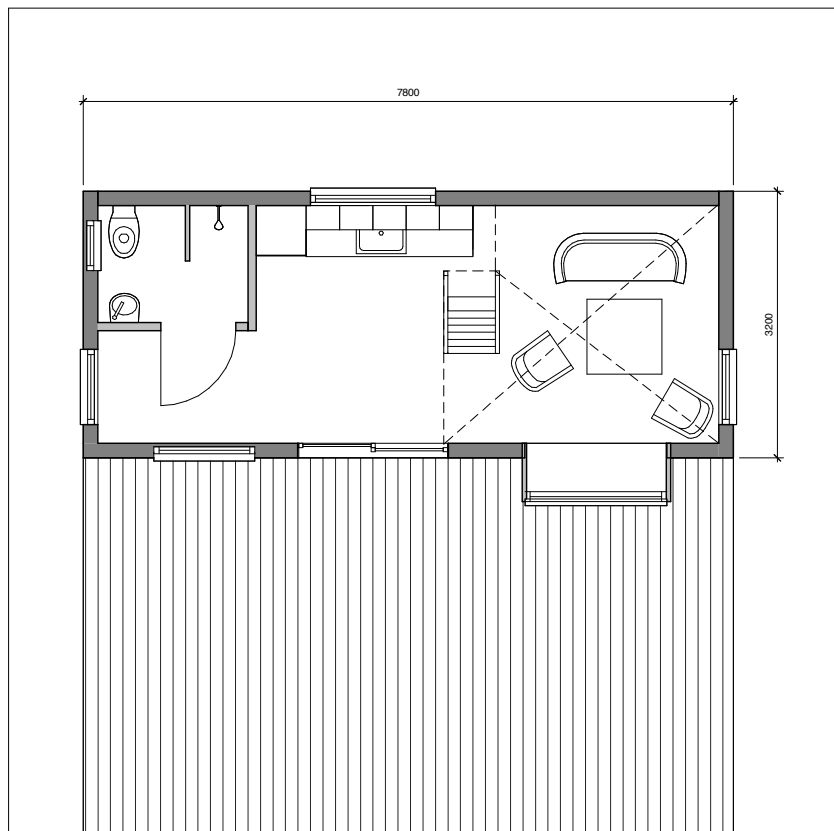
1 Plan 1 1-50 1 : 50
